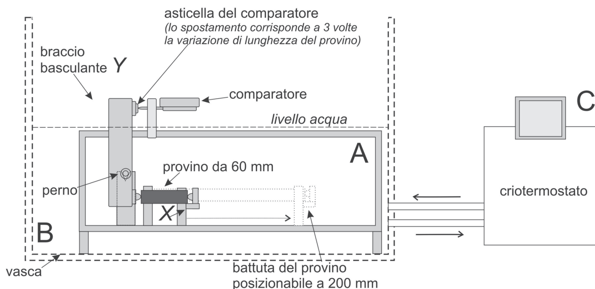
Fig. 1 - Schema semplificato dello strumento proposto per misurare la dilatazione idrica lineare conseguente all'assorbimento d'acqua per immersione totale. A = dilatometro; B = recipiente contenente acqua alla temperatura di misura ( T = 20^\circ\text{C} ) nel quale sono immersi il campione ed il dilatometro; C = criotermostato; X = supporti portacampione; Y = braccio basculante che collega il campione al comparatore digitale.
