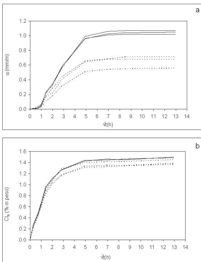
Fig. 4 - a) Curve di dilatazione idrica lineare ( \alpha , mm/m) in funzione della radice quadrata del tempo di provini di un campione di arenaria Macigno, misurati perpendicolarmente (tratto continuo) e parallelamente (tratteggiato) al verso della roccia; b) Curve di assorbimento d'acqua per immersione totale ( C_{IP} , % in peso) in funzione della radice quadrata del tempo, relative ai provini di Figura 4a.
