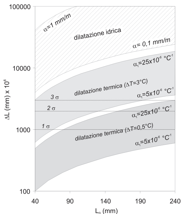
Fig. 3 - Valore della variazione di lunghezza ( \Delta L , mm) in funzione della lunghezza iniziale ( L_0 , mm) dei campioni, per valori della dilatazione idrica ( \alpha , mm/m) e della dilatazione termica ( \alpha_t , ^\circ\text{C}^{-1} ) corrispondenti a quelli presentati dalle rocce più comuni. La dilatazione termica è riportata per \Delta T = 0,5^\circ\text{C} e \Delta T = 3^\circ\text{C} . Le linee orizzontali tratteggiate corrispondono all'errore strumentale del comparatore digitale impiegato per effettuare le misure di dilatazione.
